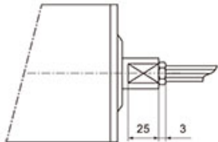
直式出线 Straight outlet
